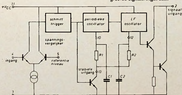
Fig. 1 a. Blokschema van het geïntegreerde signaleringcircuit.
